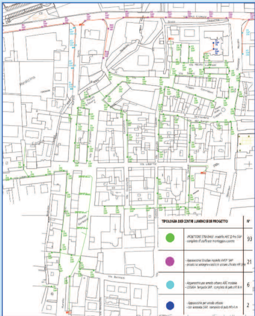
Sopra: la mappa dell'area del centro storico oggetto di intervento con l'indicazione delle nuove linee e punti luce. Sotto: due immagini delle linee aeree del centro storico. A destra il lampione AEC modello Logika previsto in via Saffi e via Mazzini.
